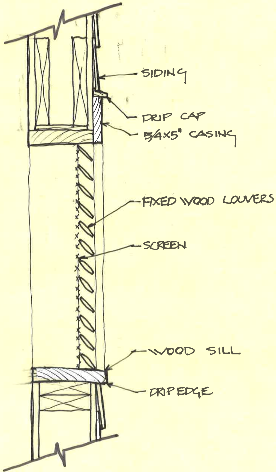
WOOD GABLE VENT N.T.S.
